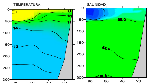
Figura 10. Distribución de a) Temperatura (°C), b) Salinidad. Sección Punta Bermejo
