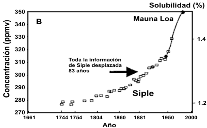
(a) Datos originales de Siple sin suponer una edad 83 años más joven para el aire que la edad del hielo que lo encierra.
