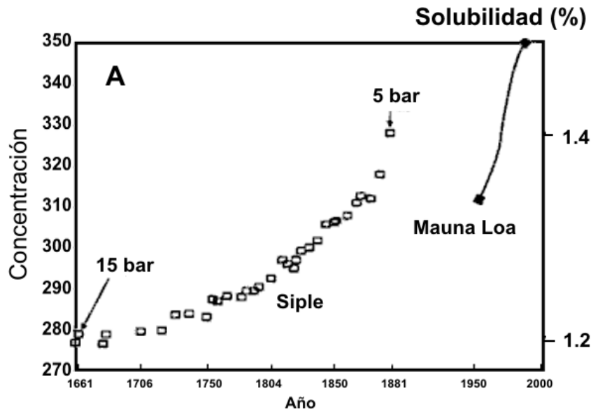
Figura 1A: Concentración de \text{CO}_2 en las burbujas de aire de hielo pre-industrial extraído en Siple, Antártida (cuadrados blancos) y de la atmósfera de Monte Mauna Loa, Hawaii 1958-1986 (línea sólida):
