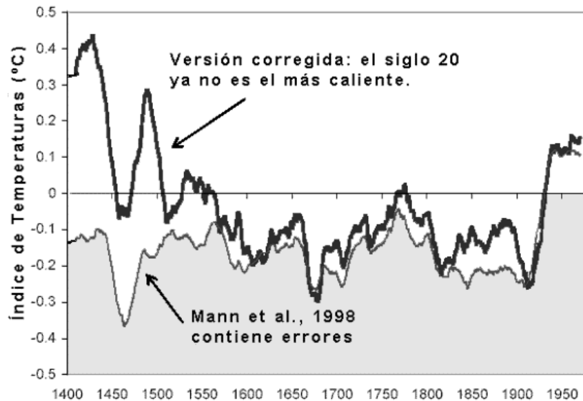
Figura 6: El Palo de Hockey rectificado por McIntyre y McKittrick
