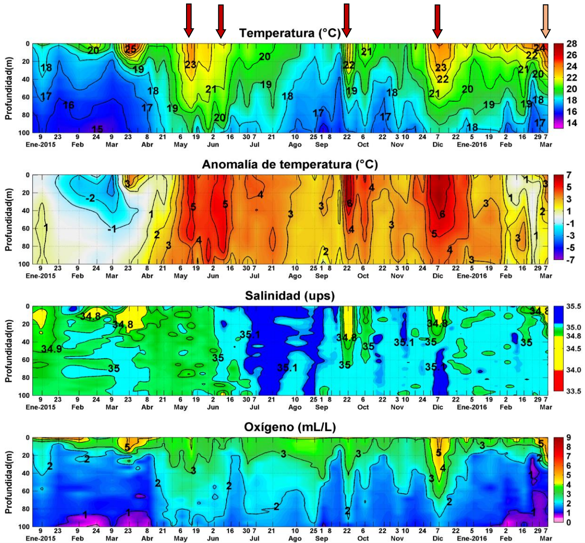
Figura 1. Series de tiempo oceanográficas en la Estación Fija Paita del IMARPE, actualizada al 7 de marzo. Las flechas rojas indican el impacto de ondas Kelvin cálidas más intensas desde enero 2015. Nótese la profundización de las isotermas (capas de similar temperatura) registrada el 7 de marzo. El rango de salinidad detectado encima de los 20 m en la última fecha corresponde a la presencia de Aguas Ecuatoriales Superficiales provenientes del norte.
