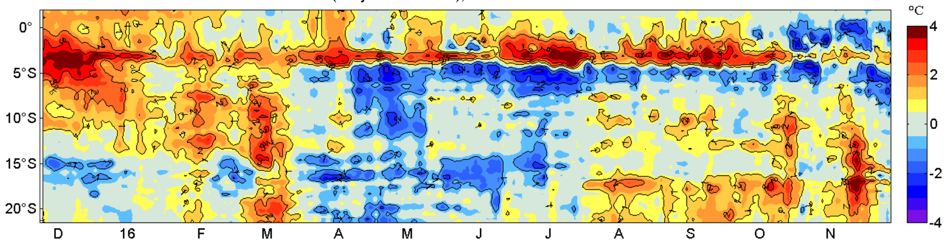
ATSM (franja ~ 0 a 50 mn), Actualizado al 28-Nov-2016
