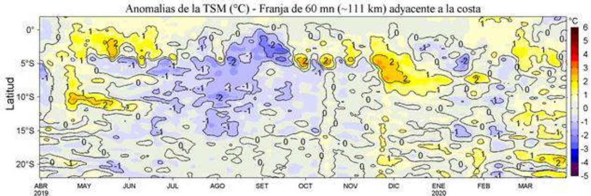
Figura 13 Diagrama Hovmöller de la anomalía de la temperatura superficial del mar frente a la costa peruana. Fuente: OSTIA (Donlon et al., 2012; UK Met Office, 2012). Producto: OSTIA-UKMO-L4-GLOB-v2.0. Procesamiento: LHFH/AFIOF/DGIOCC/IMARPE.
