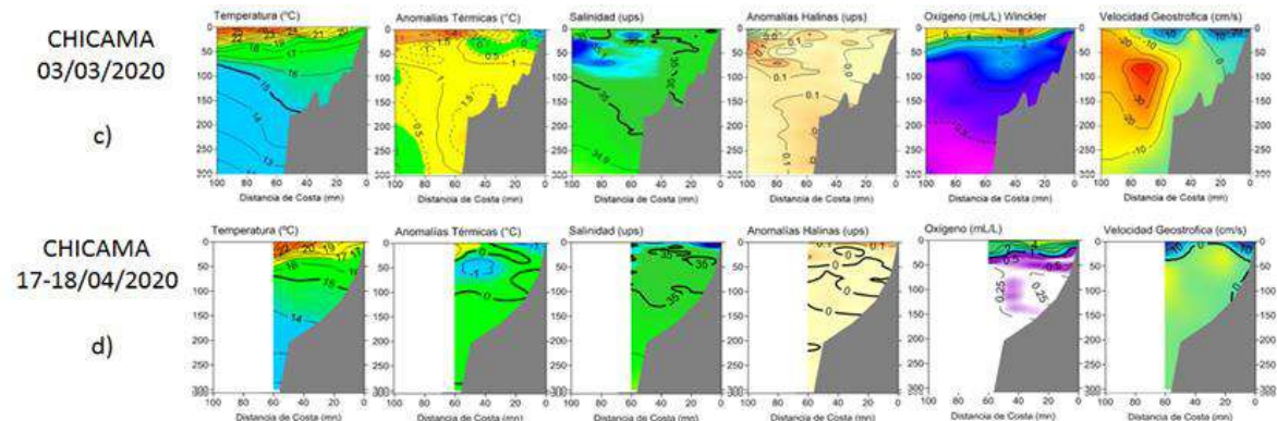
Figura 19 Distribución vertical de temperatura ( ^{\circ}\text{C} ), anomalía térmica ( ^{\circ}\text{C} ), salinidad (ups), anomalía halina (ups), oxígeno disuelto (mL/L) y corrientes geostroficas en el perfil Chicama.
