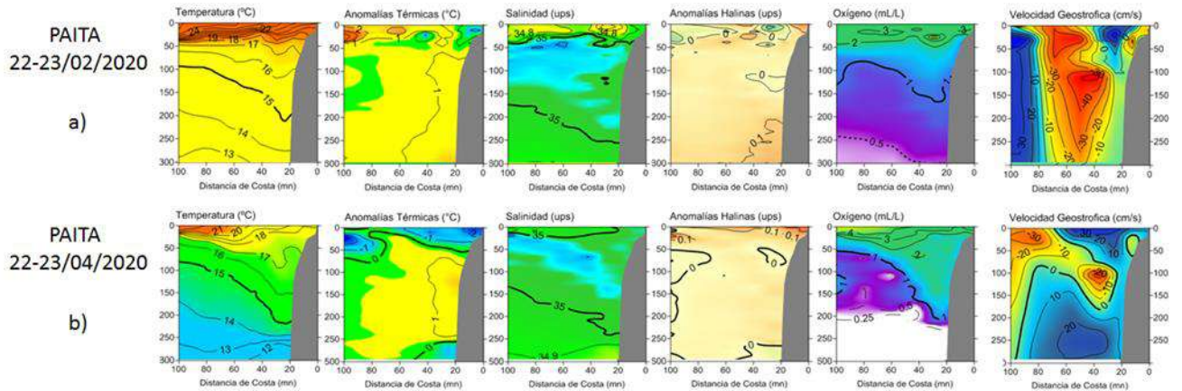
Figura 18 Distribución vertical de temperatura (°C), anomalía térmica (°C), salinidad (ups), anomalía halina (ups), oxígeno disuelto (mL/L) y corrientes geostroficas en el perfil Paíta.
