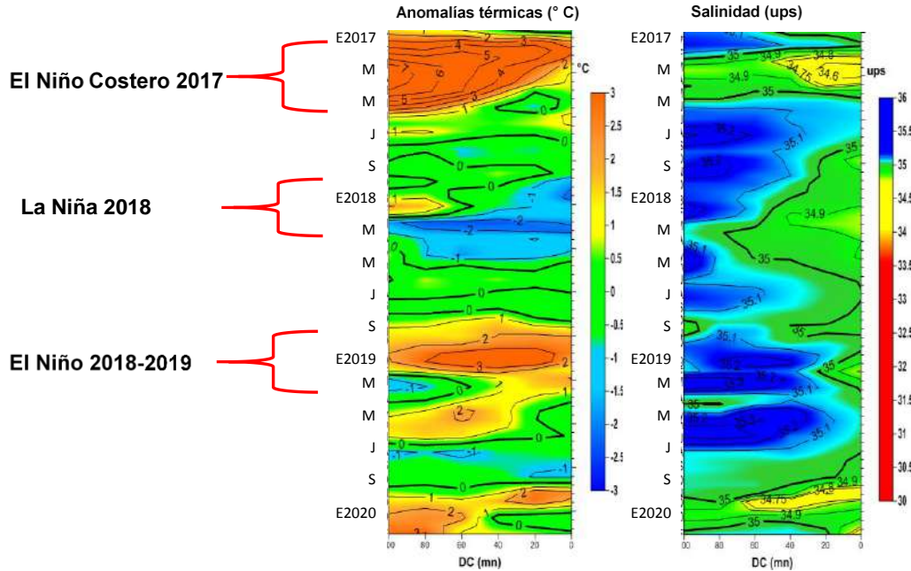
Figura 17 Diagramas Hovmöller de la distribución de la a) ATSM y b) SSM frente a Chicama, para el periodo 2017 al 2020 y entre la costa y las 100mn.
